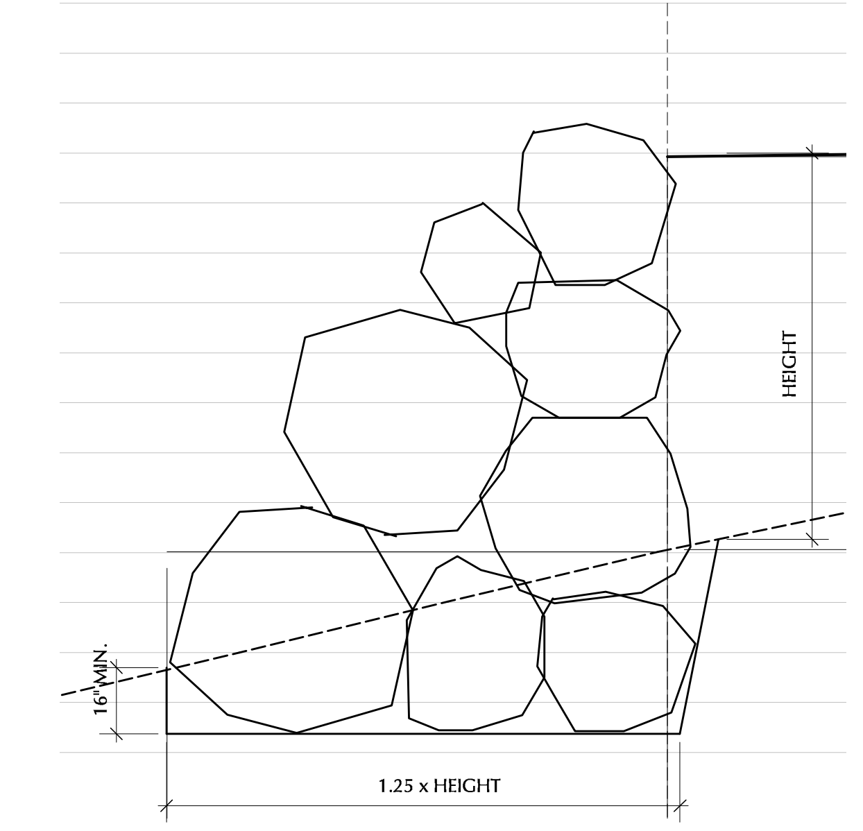
3 C-6 DETAIL Scale: 3/8" = 1'-0"
